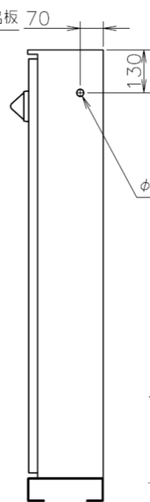
側面図
