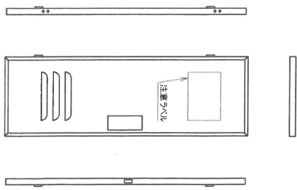
扉背面図
